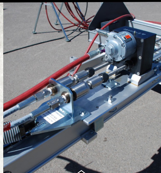
Giunti SL montati su lancia
