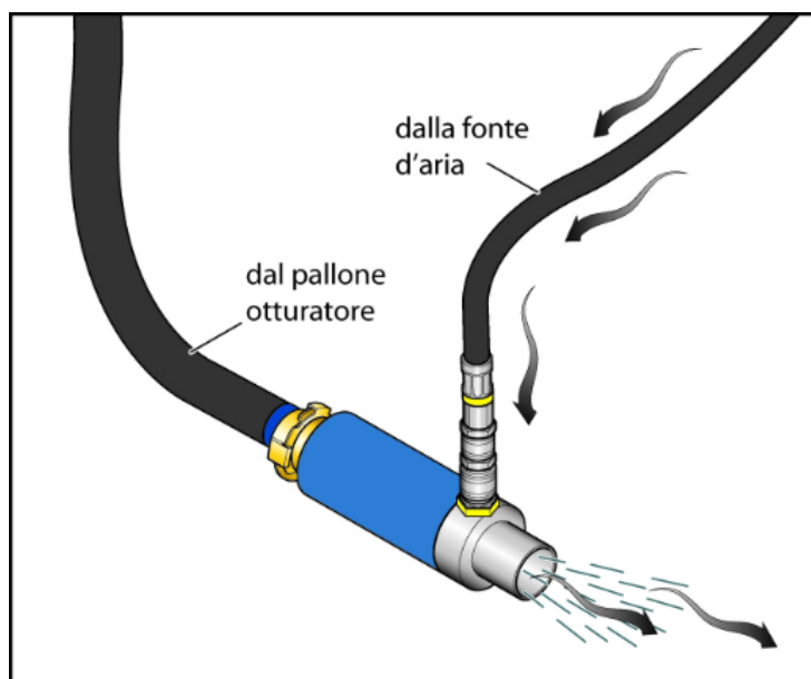
Figura 1 – Eiettore.
